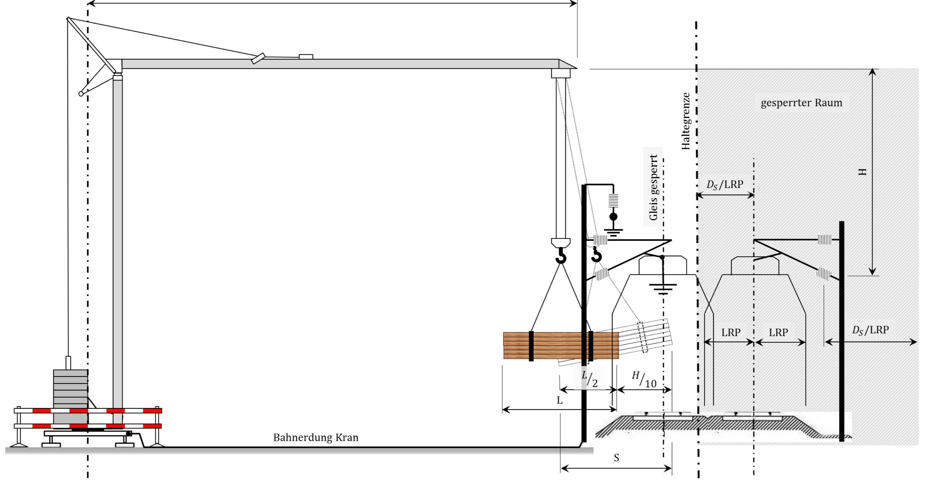
Situation III – Sicherheit durch Abschränkung / Schutzwand
