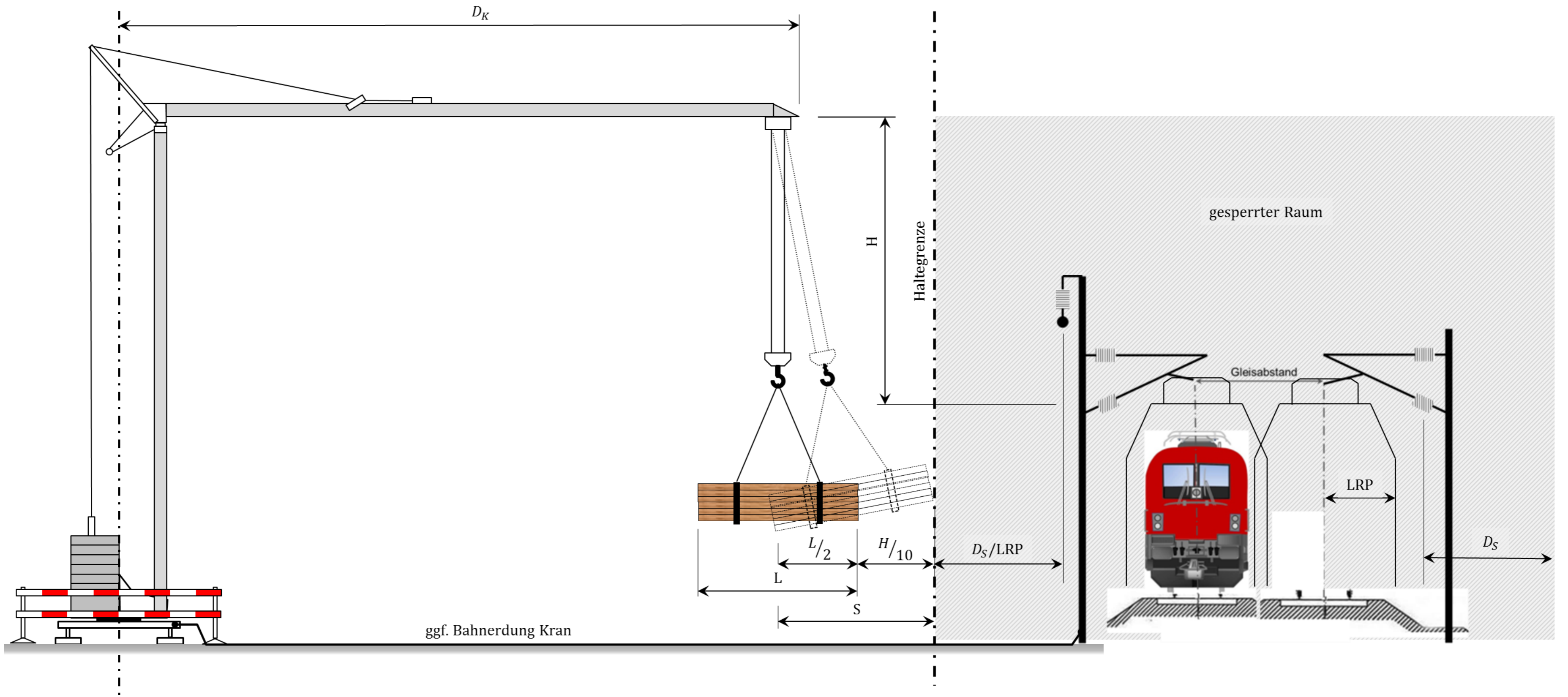
Situation I – Sicherheit durch Abstand
