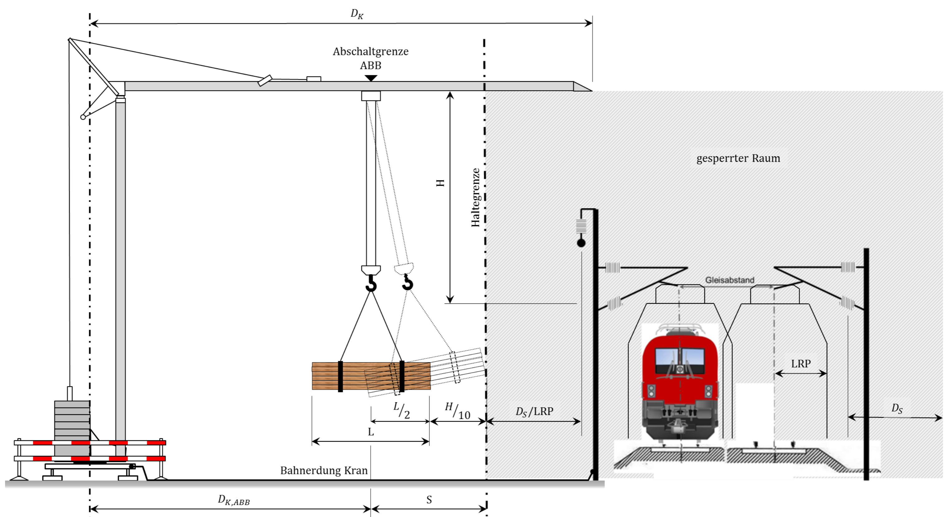
Situation II – Sicherheit durch Abstand und ABB
