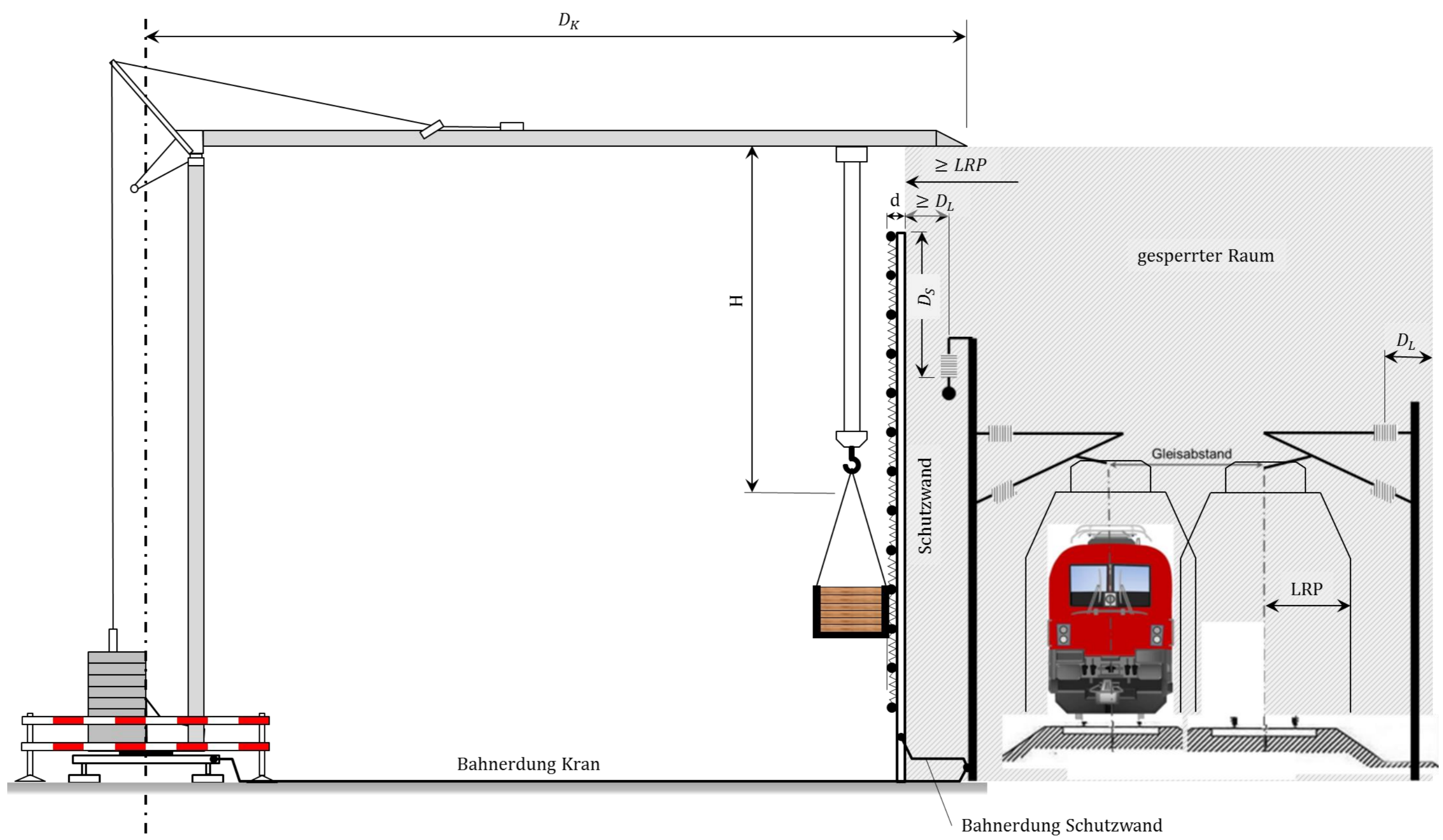
Situation III – Sicherheit durch Abschränkung / Schutzwand
