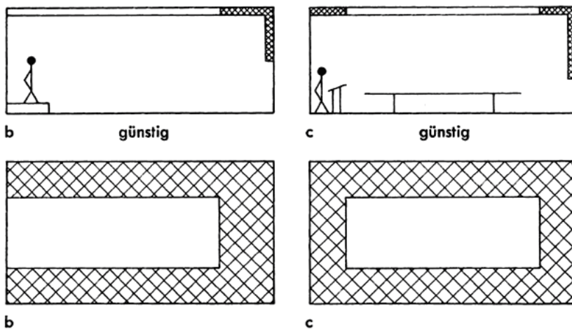
Bild 1: Verteilung von Schallabsorptionsflächen (schraffierte Flächen) in Unterrichtsräumen, jeweils im Aufriss und als Deckenuntersicht (Quelle: DIN 18041).
