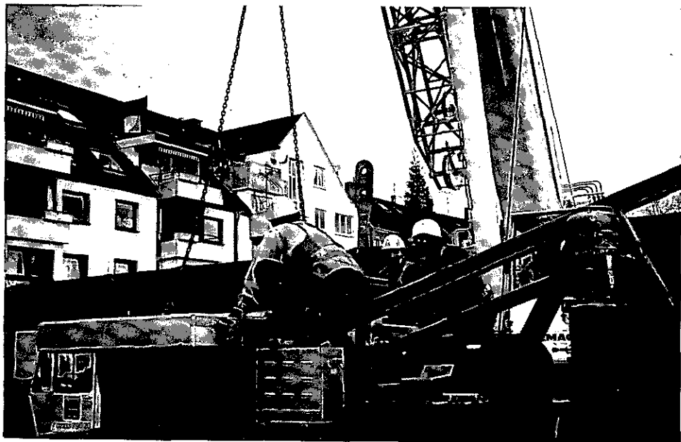
Abbildung 21: Turmdrehkranaufstellung (B 58, B 59, B 60)
