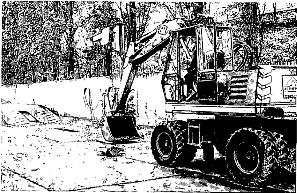
Abbildung 15: Baggergreifer wechseln (B 36)
