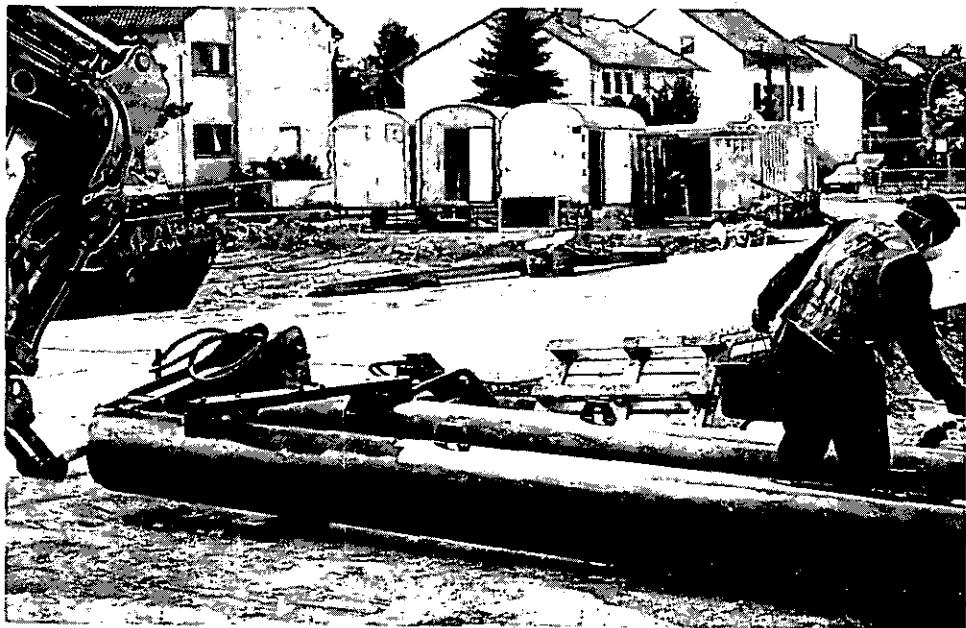
Abbildung 14: Auftriebskörper für Schwimmbagger schweißen (B 33)
