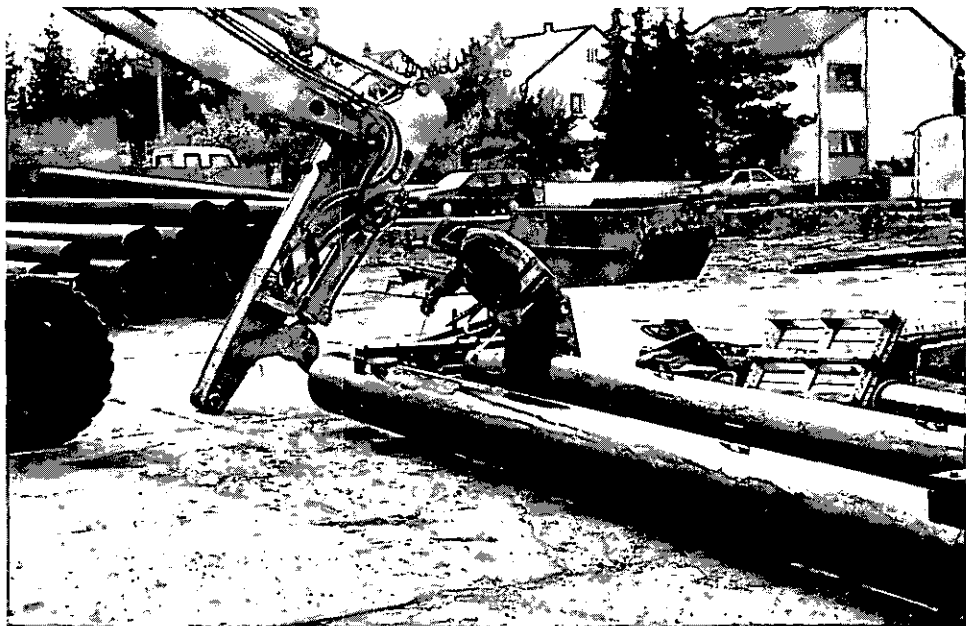
Abbildung 16: Pontone fertigstellen (B 37)
